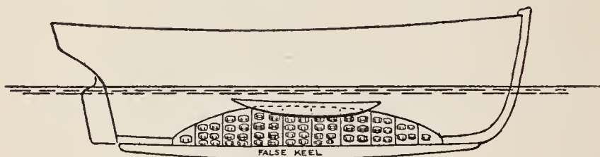
SLOOP "LUCY" 1828.
