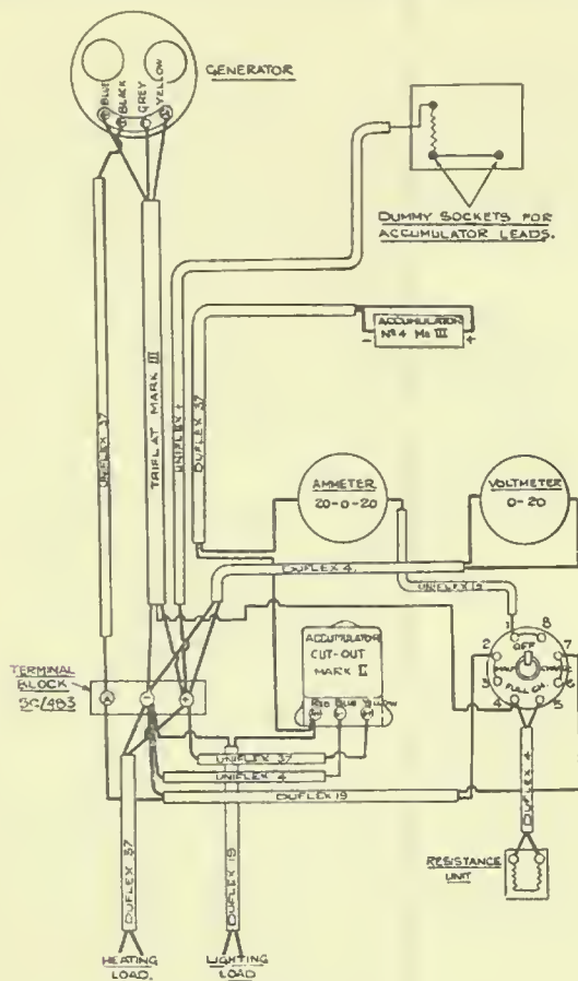
WIRING DIAGRAM.
