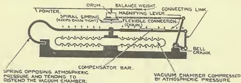
FIG. 61. ANEROID ALTIMETER
