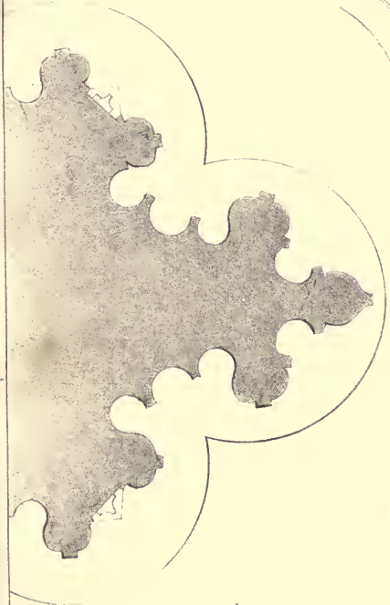
Mouldings of Archivolts 1 1/2 inch Scale to one foot
