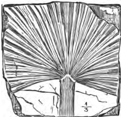
PALMACITES LAMANONIS.
