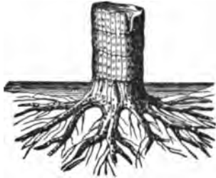
SIGILLARIA RENIFORMIS.
