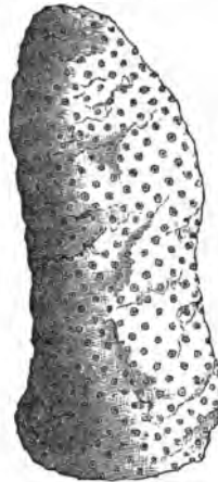
STIGMARIA.
