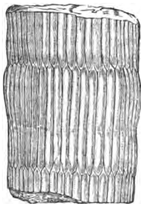
EQUISETUM COLUMNARE.
