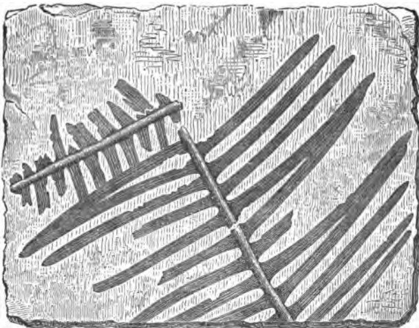
PHLEBOPTERIS.
