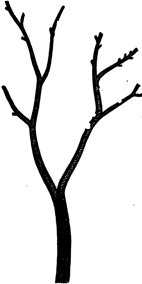
LEPIDODENDRON STERNBERGII.
