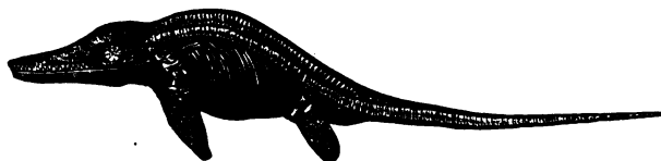
ICHTHYOSAURUS COMMUNIS. (Lias.)
