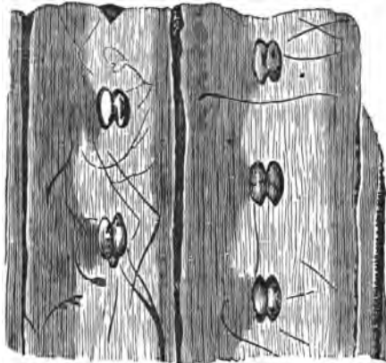
SIGILLARIA RENIFORMIS.
