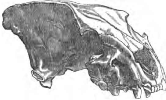
HYÆNA SPELÆA. Cave Hyæna. ( Pleistocene. )
