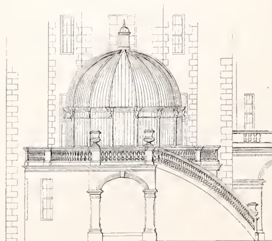
END ELEVATION
