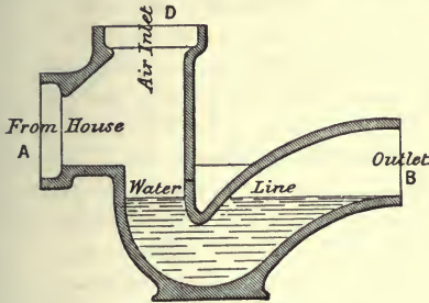
Fig. 283.—Ventilating Trap.
