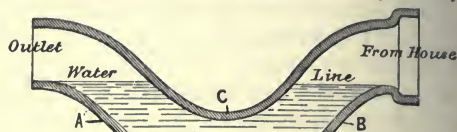
Fig. 281.—Syphon Trap.
